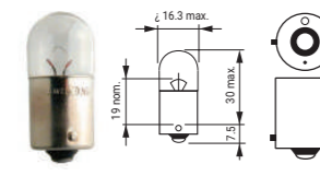
10 R5W BASE BA15s
