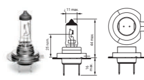
3 H7 BASE PX26d
